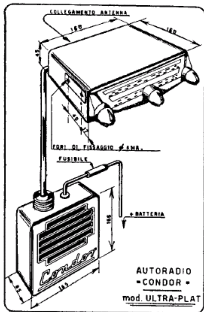
Fig. 26.19. - Autoradio CONDOR Mod. ULTRA-PLAT. Sistemazione dell'impianto.
